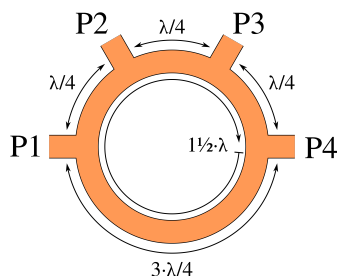
Abbildung 1. Struktur eines konventionellen Rat-Race-Kopplers gemäß [3]
