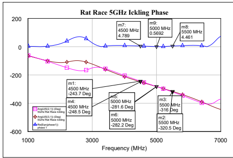
Abbildung 6. Simulierter Phasenverlauf des Rat-Race-Kopplers bei 5 GHz
