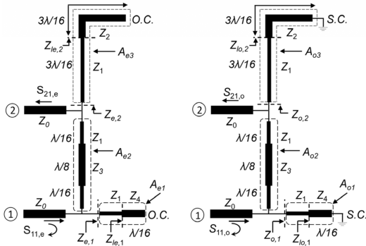
Abbildung 3. Leitungslängen aus der Literatur [1].
