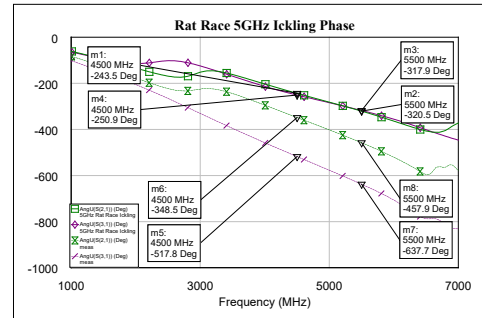
Abbildung 10. Vergleich des simulierten und gemessenen Phasenverlaufs
