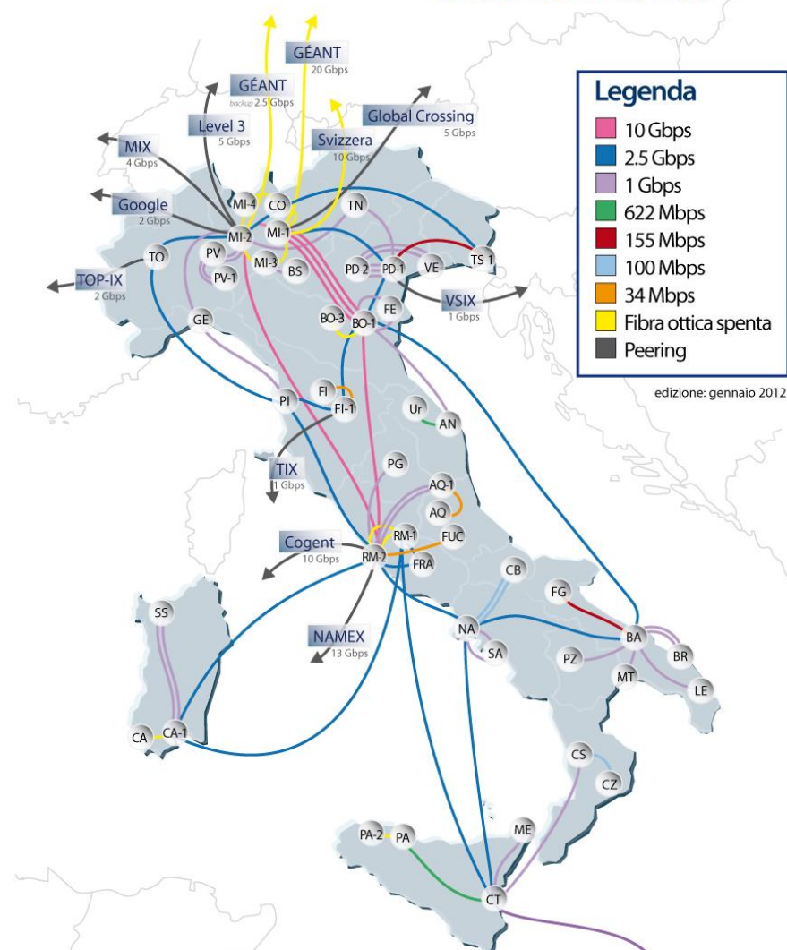
Topologia di backbone della rete GARR
