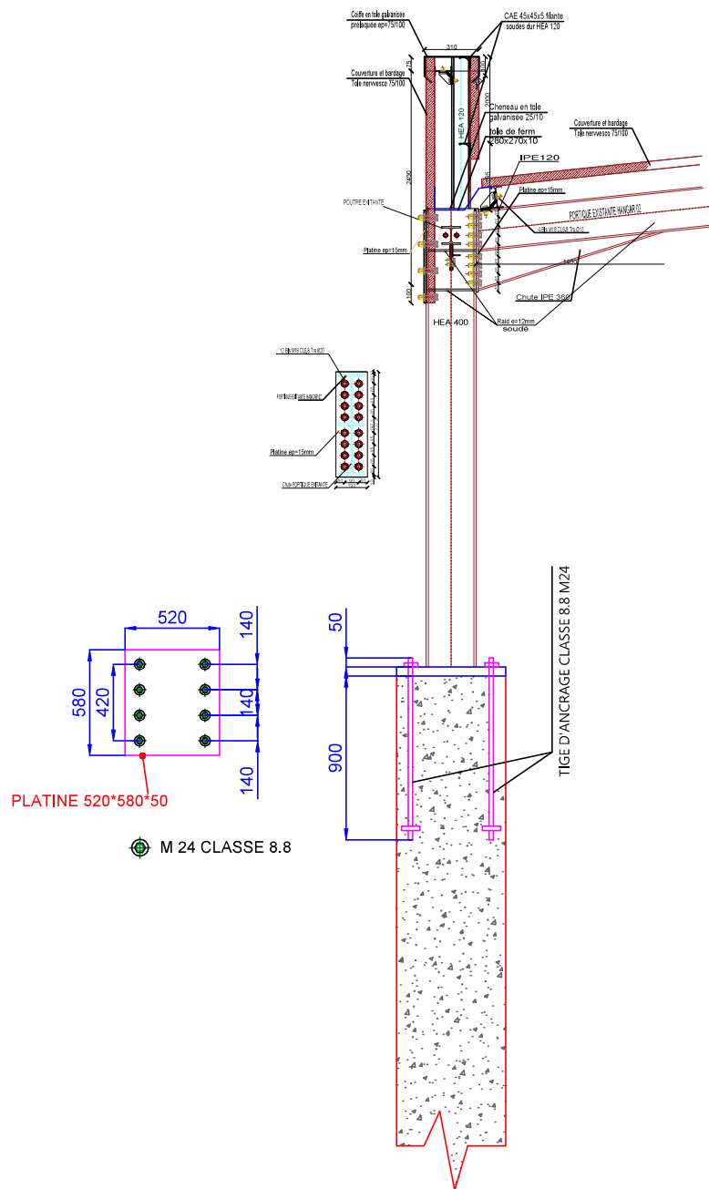
DETAIL N01 VUE A-A HANGAR 02
