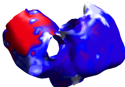
Cons-Tikh
