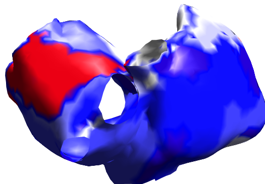
Tikh
