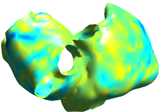
Tikh
