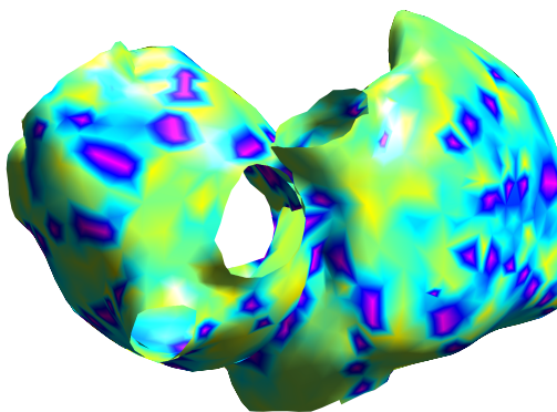
Cons-Tikh
