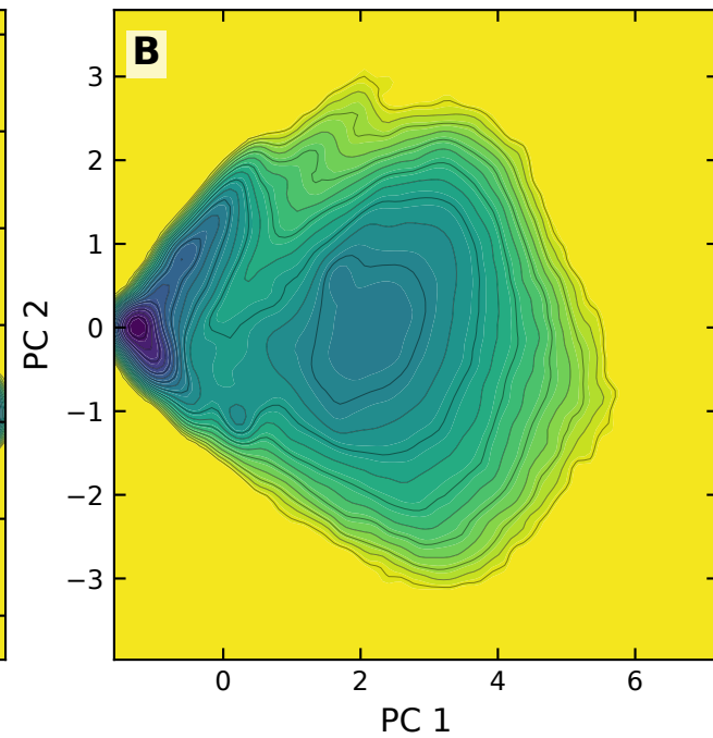
PCA distances
