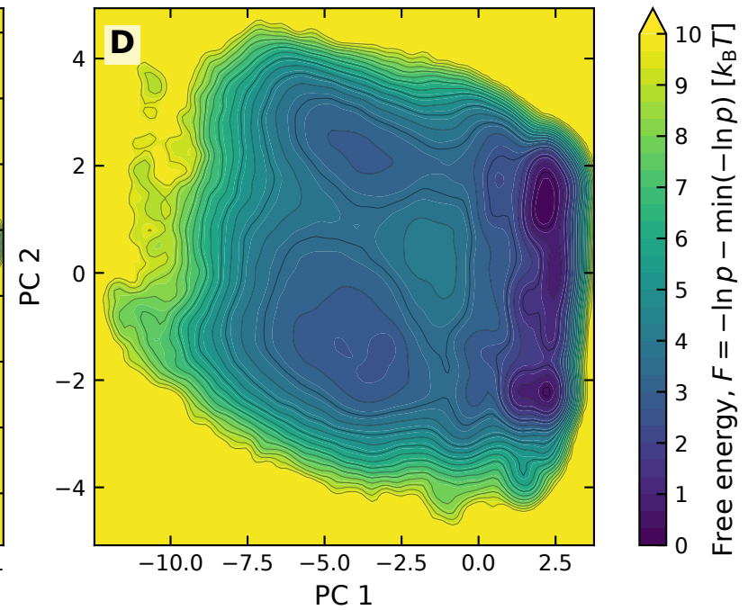
PCA dihedrals
