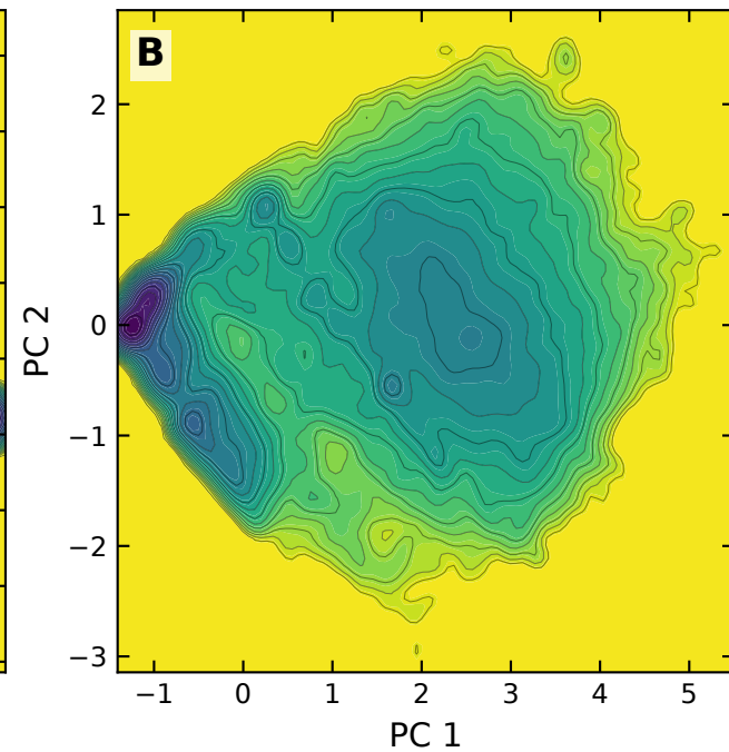
PCA distances
