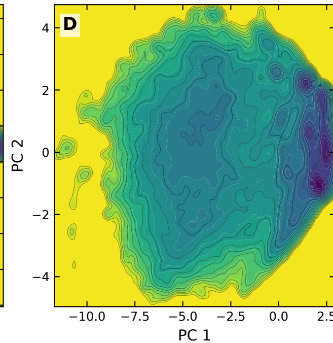
PCA dihedrals
