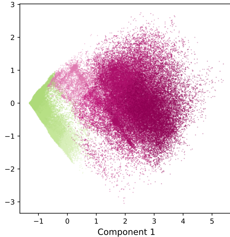
pca distances
