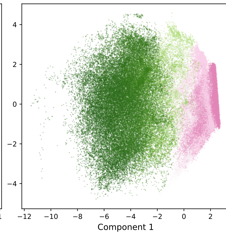
pca dihedrals
