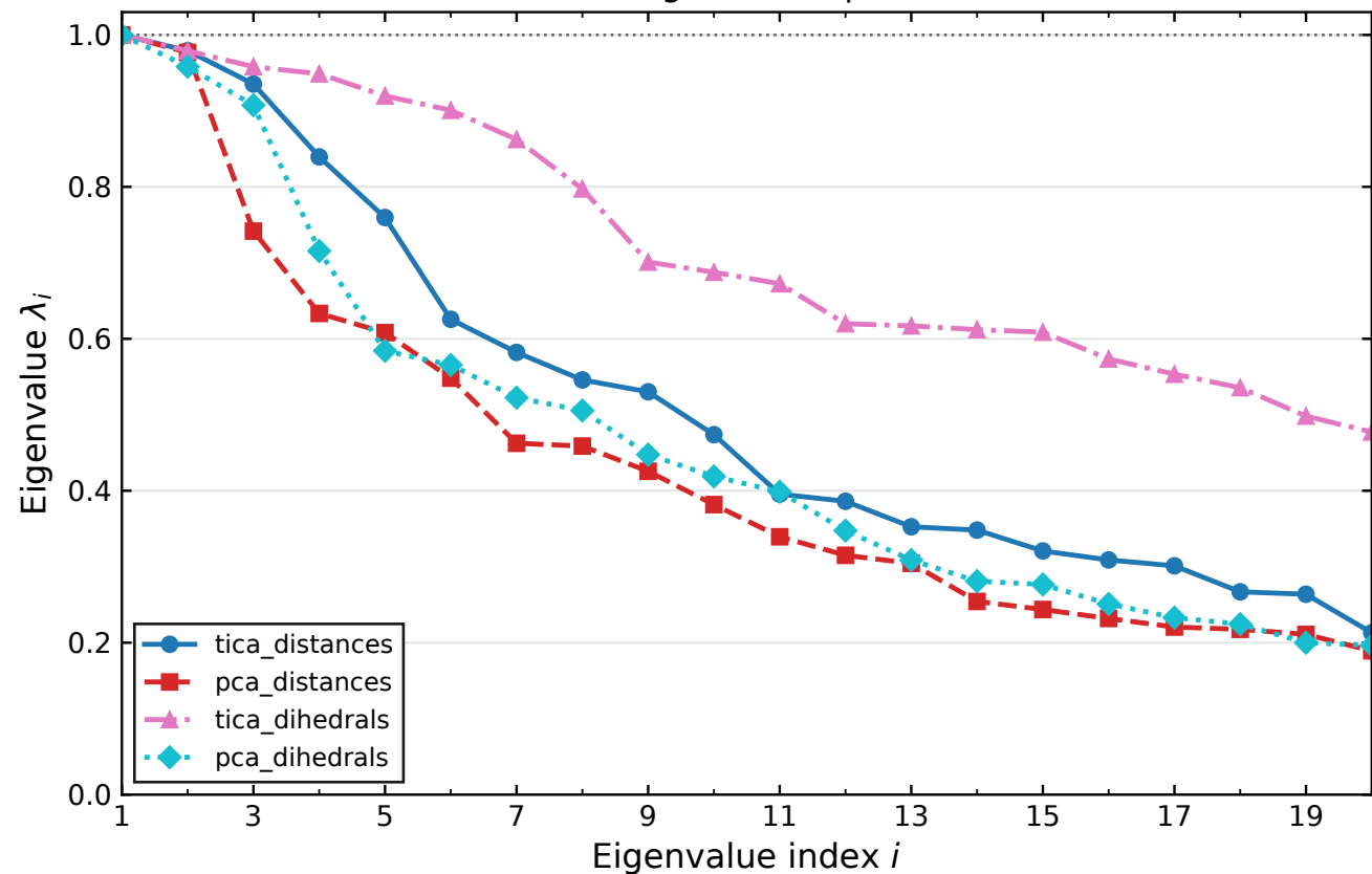
MSM eigenvalue spectra
