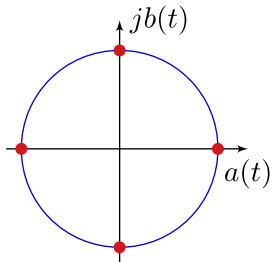
2^2 -wertiges PSK-Signal (QPSK)
