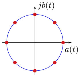
2^3 -wertiges PSK-Signal (8-PSK)
