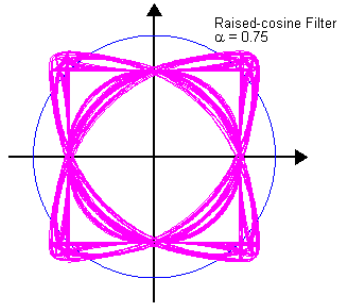
Offset QPSK mit \alpha = 0.75
