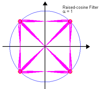
QPSK mit \alpha = 1
