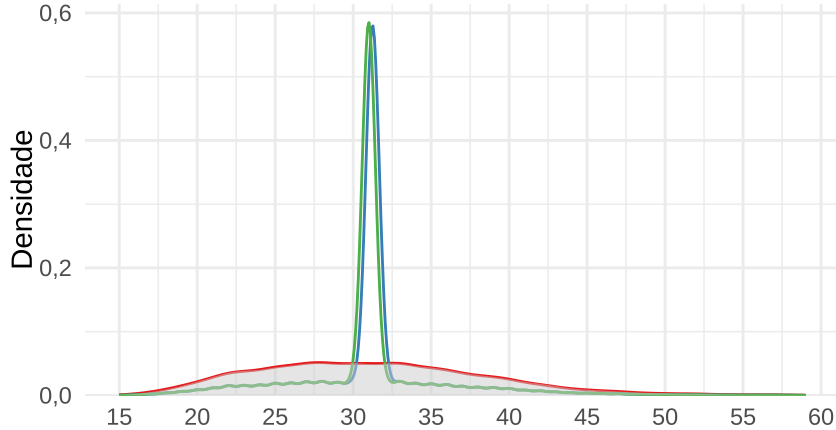
MNAR
