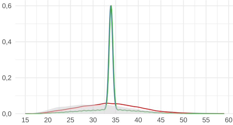
MCAR
