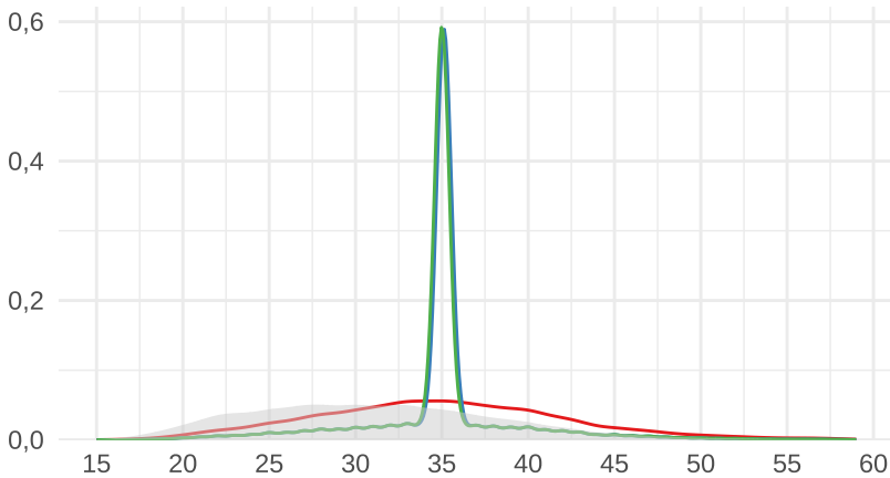
MNAR
