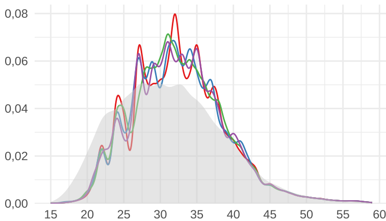
MNAR
