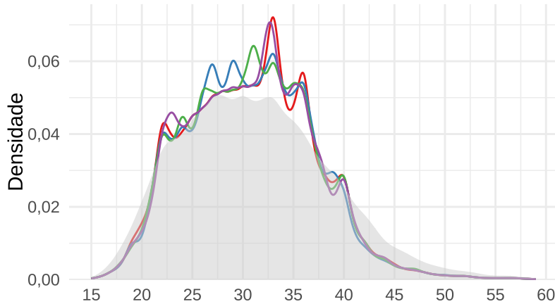
MNAR
