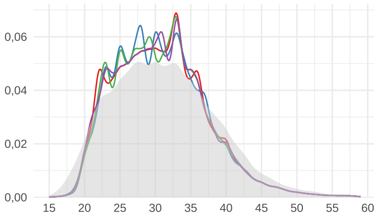
MCAR
