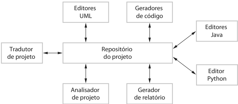
Figura 6.6 Uma arquitetura de repositório para um IDE
