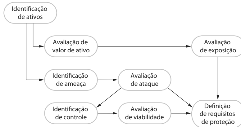
Figura 12.4 O processo de avaliação preliminar de riscos para requisitos de proteção
