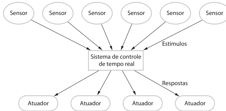
Figura 20.1 O modelo geral de sistemas embutidos de tempo real
