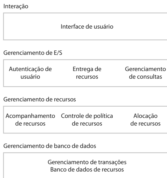
Figura 16.4 A arquitetura de um sistema de alocação de recursos
