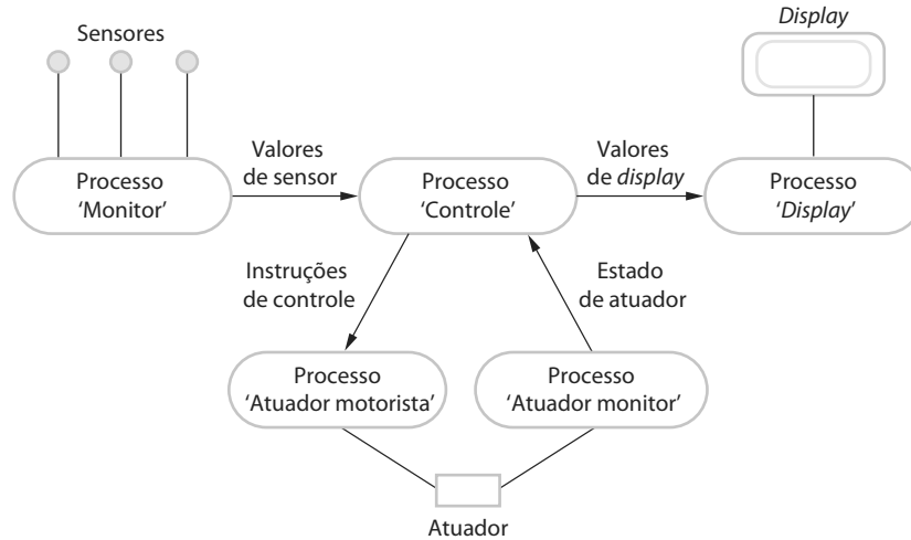
Figura 20.7 Estrutura de processo 'Controle de ambiente'
