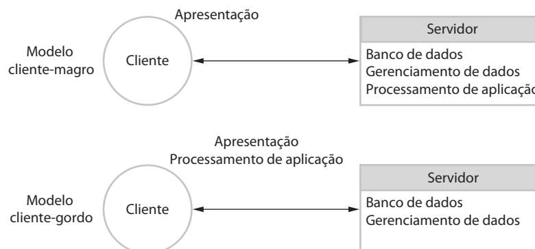
Figura 18.7 Modelos de arquitetura cliente-magro e cliente-gordo
