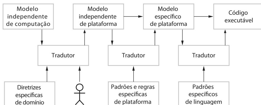
Figura 5.17 Transformações de MDA
