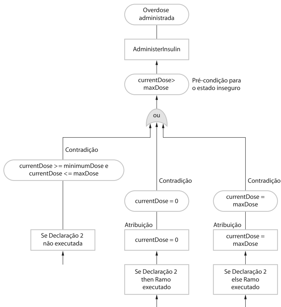
Figura 15.6 Argumento informal de segurança baseado em demonstrações de contradições
