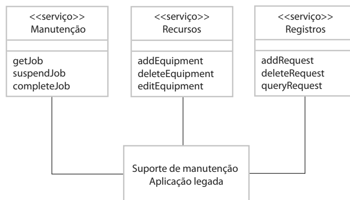
Figura 19.7 Serviços fornecendo acesso a um sistema legado
