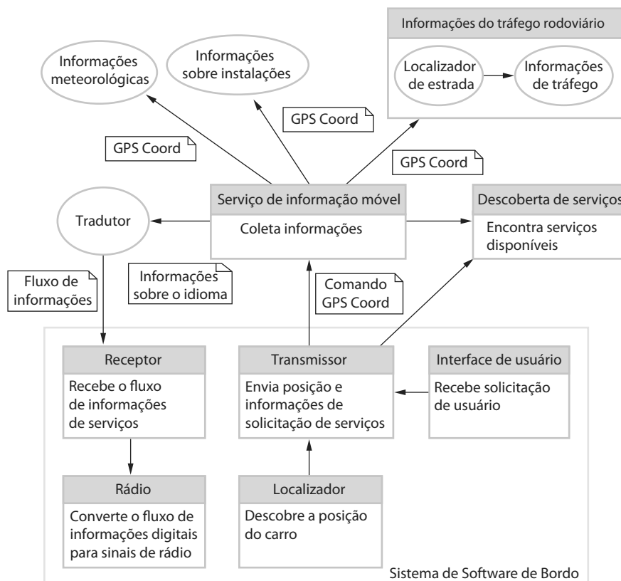
Figura 19.3 Um sistema de informações de bordo baseado em serviços
