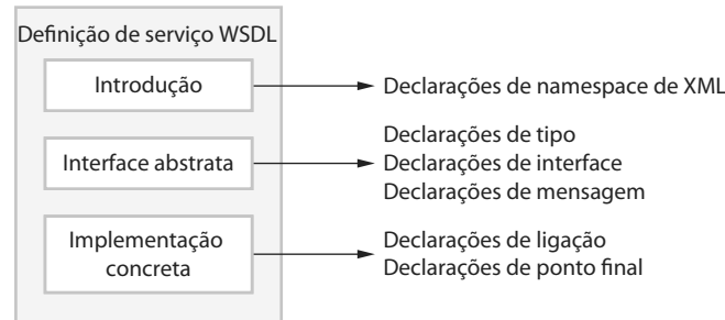
Figura 19.4 A organização de uma especificação WSDL
