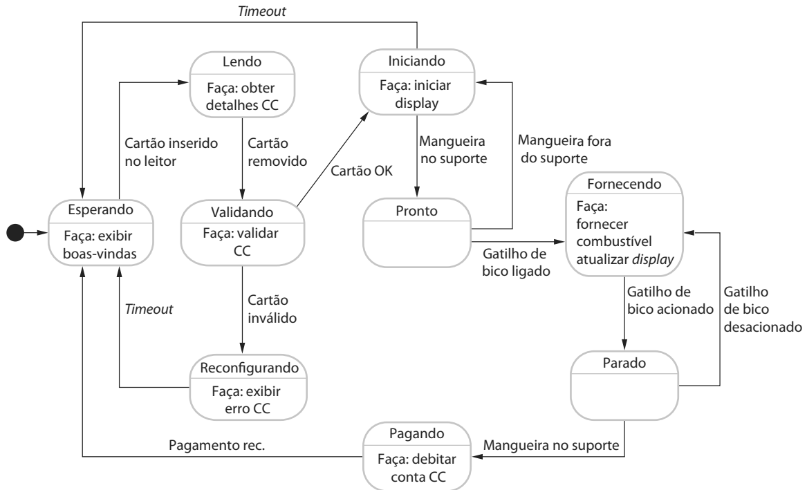
Figura 20.4 Modelo de máquina de estado de uma bomba de gasolina
