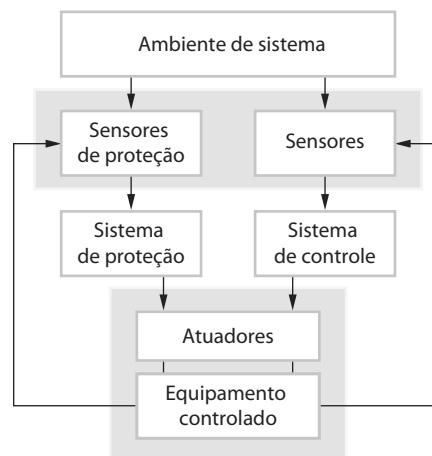
Figura 13.2 Arquitetura de sistema de proteção
