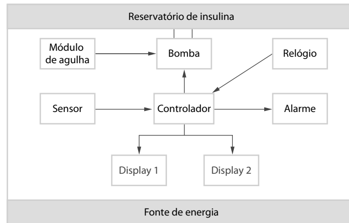
Figura 1.1 Hardware de bomba de insulina
