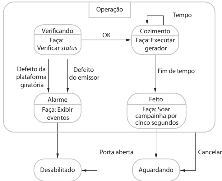
Figura 5.16 Operação do forno de micro-ondas
