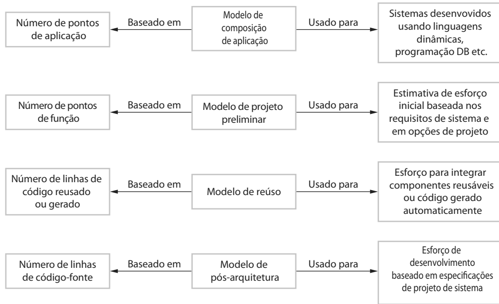
Figura 23.7 Modelos de estimativa COCOMO
