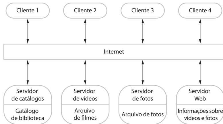
Figura 6.7 Uma arquitetura cliente-servidor para uma biblioteca de filmes
