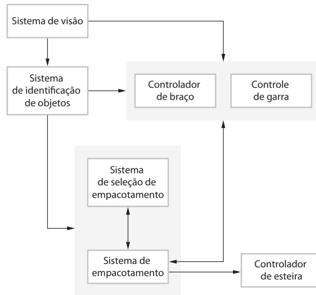
Figura 6.1 A arquitetura de um sistema de controle robotizado de empacotamento
