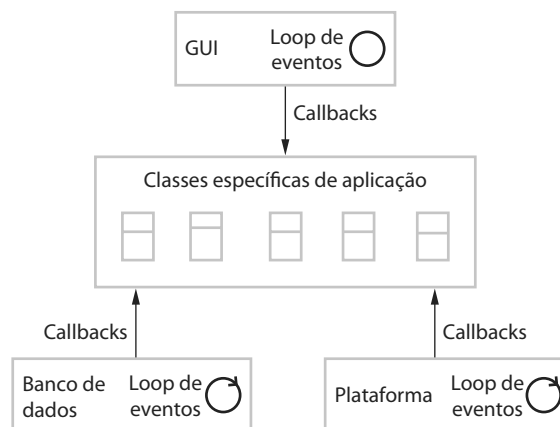
Figura 16.3 Inversão de controle em frameworks
