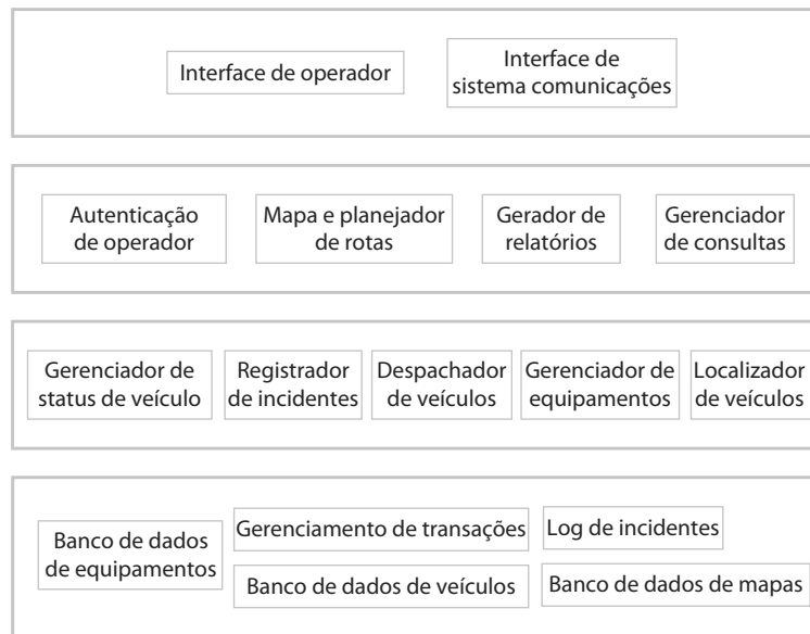
Figura 16.5 A arquitetura de linha de produto de um sistema de despacho de veículos
