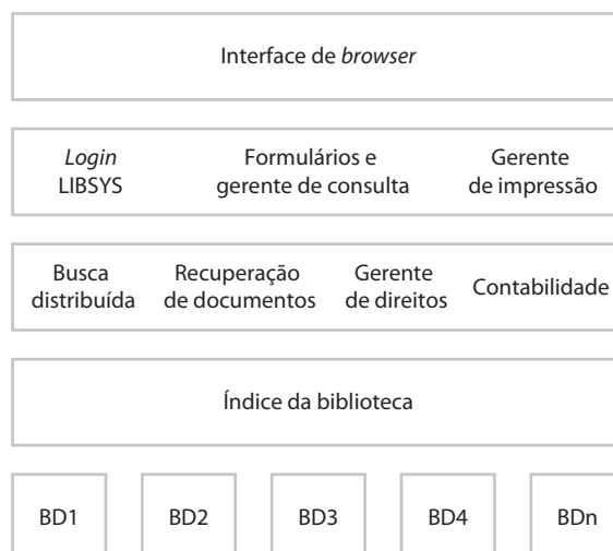
Figura 6.5 A arquitetura do sistema LIBSYS
