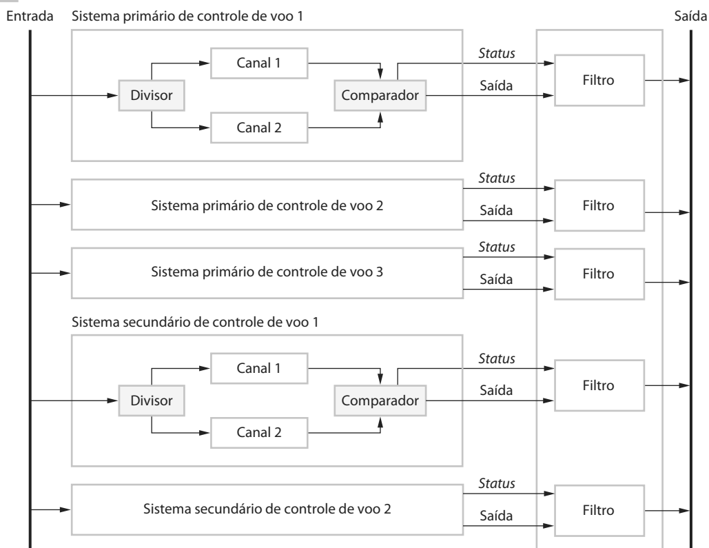
Figura 13.4 Arquitetura de controle do sistema de voo do Airbus
