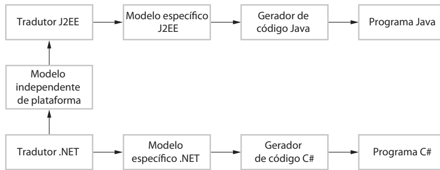
Figura 5.18 Vários modelos específicos de plataforma
