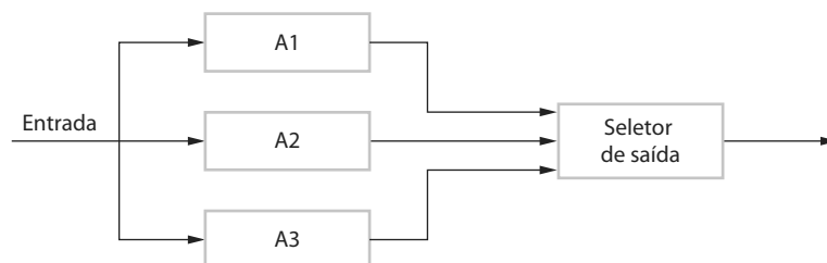
Figura 13.5 Redundância modular tripla
