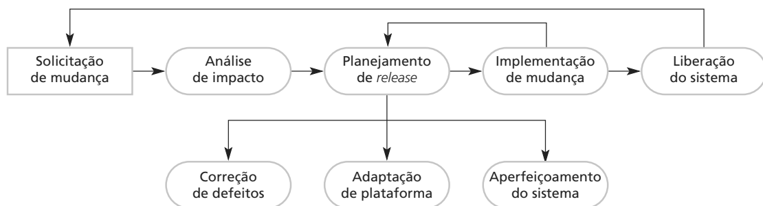
Figura 9.4 O processo de evolução de software
