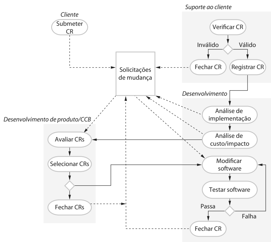
Figura 25.2 O processo de gerenciamento de mudanças
