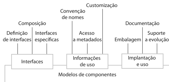
Figura 17.3 Elementos básicos de um modelo de componentes
