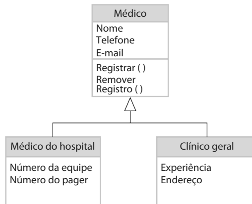
Figura 5.11 Uma hierarquia de generalização com detalhes adicionais
