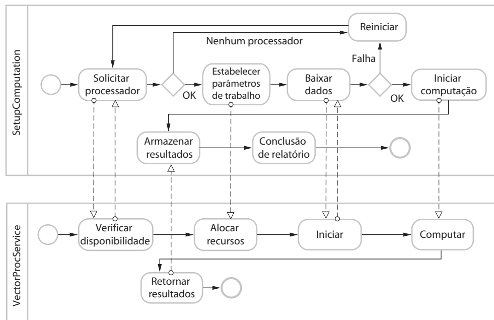
Figura 19.11 Interação de workflows
