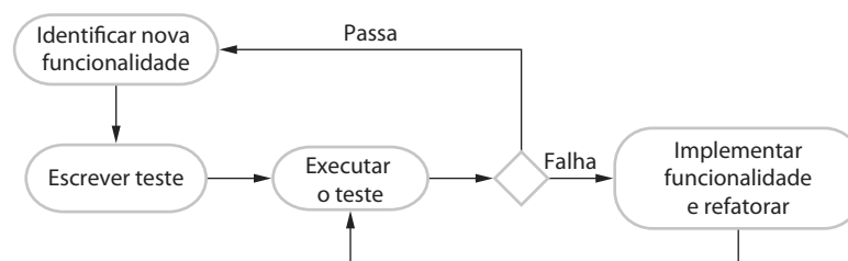
Figura 8.9 Desenvolvimento dirigido a testes
