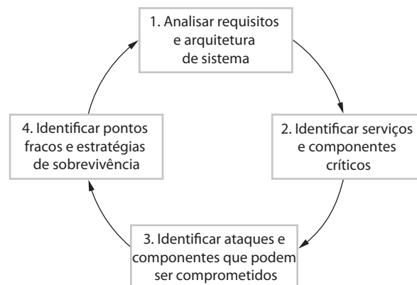
Figura 14.7 Estágios na análise de sobrevivência
