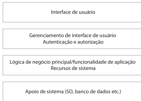
Figura 6.4 Uma arquitetura genérica em camadas
