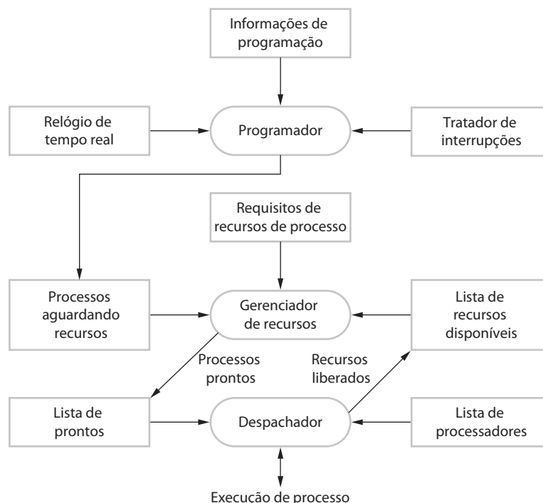
Figura 20.12 Componentes de um sistema operacional de tempo real
