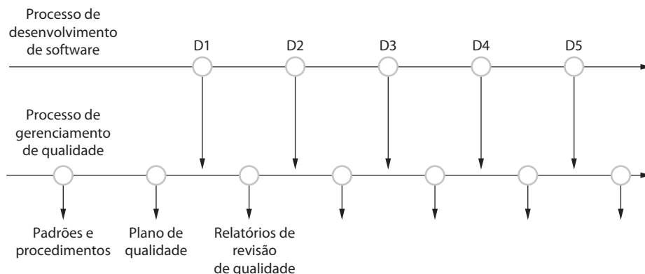
Figura 24.1 Gerenciamento de qualidade e desenvolvimento de software
