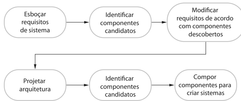
Figura 17.6 CBSE com reúso
