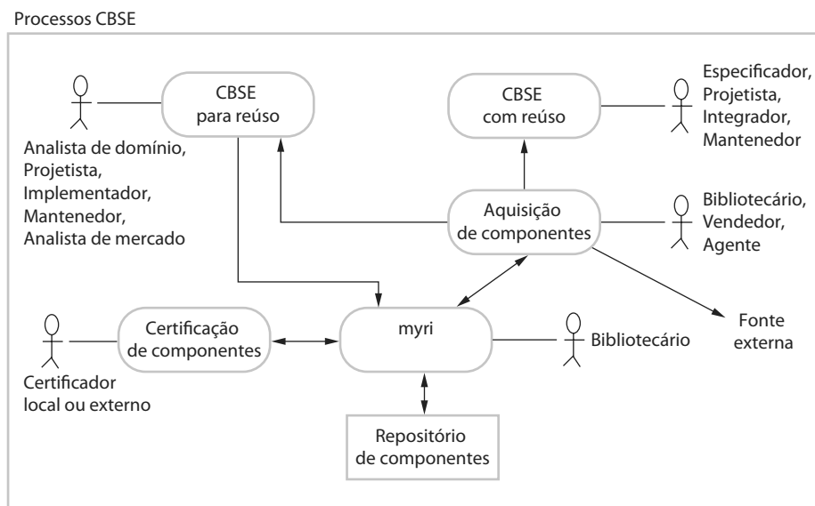
Figura 17.5 Processos CBSE
