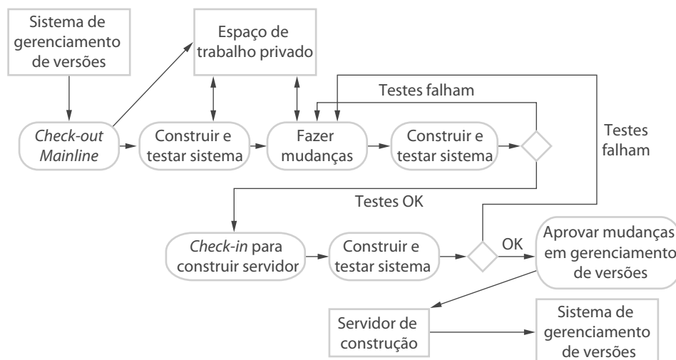
Figura 25.9 Integração contínua
