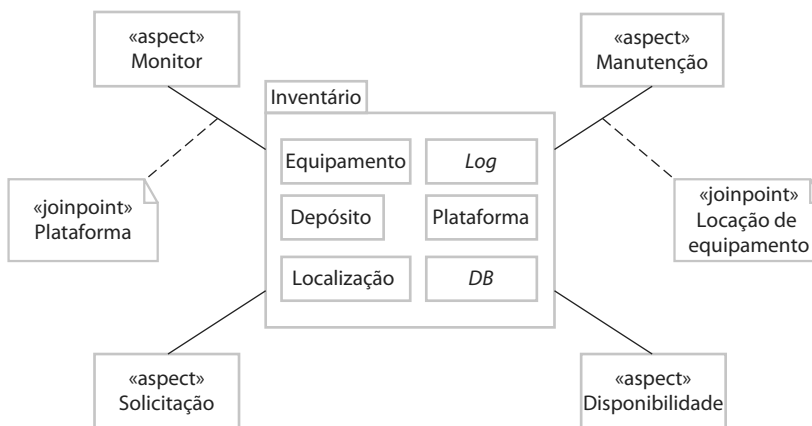
Figura 21.9 Um modelo de projeto orientado a aspectos
