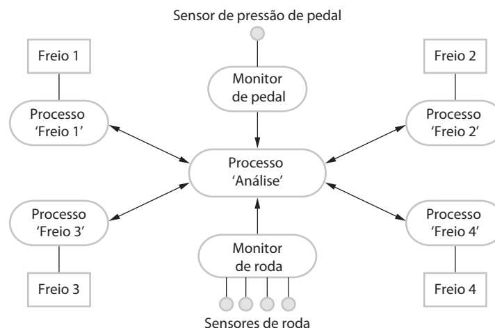
Figura 20.8 Arquitetura de sistema de controle de um sistema de frenagem antiderrapante
