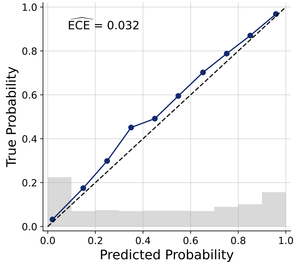
DDM
