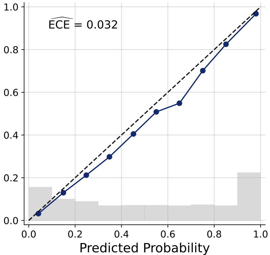
OUM
