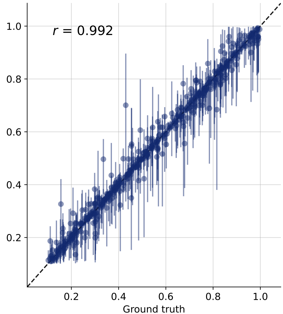
\tau (NDT)
