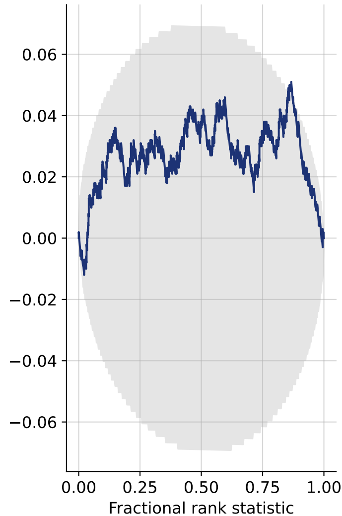
\tau (NDT)
