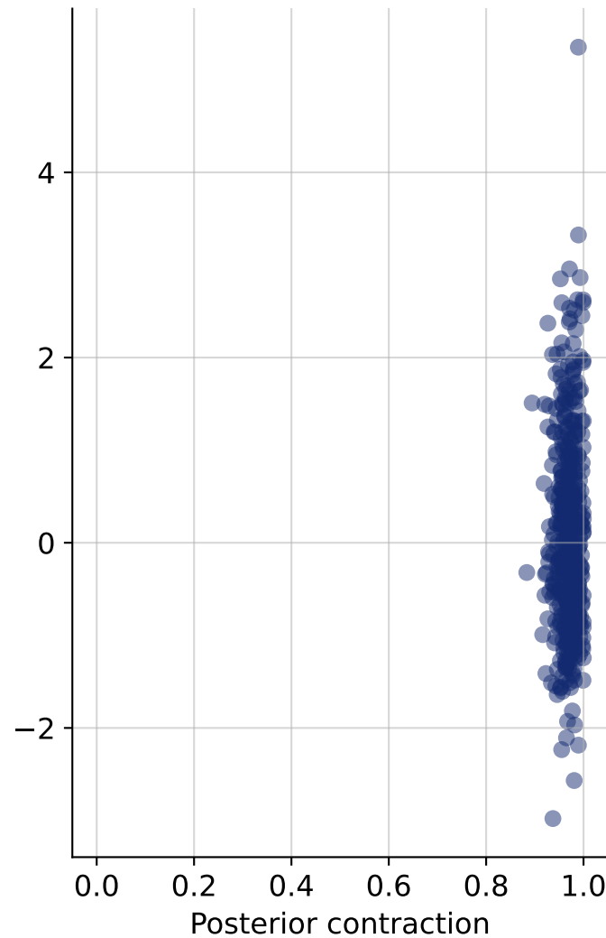
\tau (NDT)
