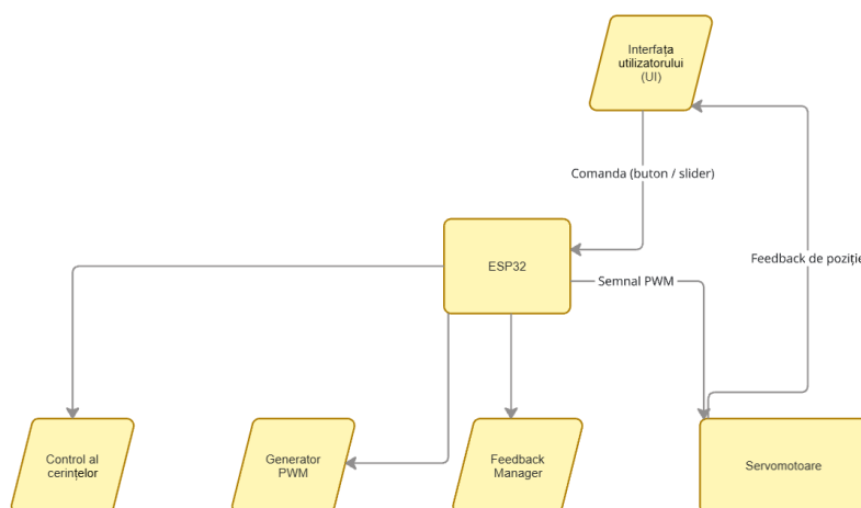
Figura 4.2. Diagrama fluxului proiectului
