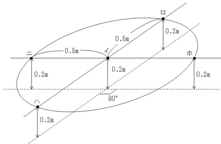
測定場所 測定方法 柱上に施設する変圧器等の下方における地表 第3項第一号により測定すること。 柱上に施設する変圧器等の周囲の建造物等 建造物の壁面等、公衆が接近することができる地点から水平方向に0.2m離れた地点において第3項第二号により測定すること。
