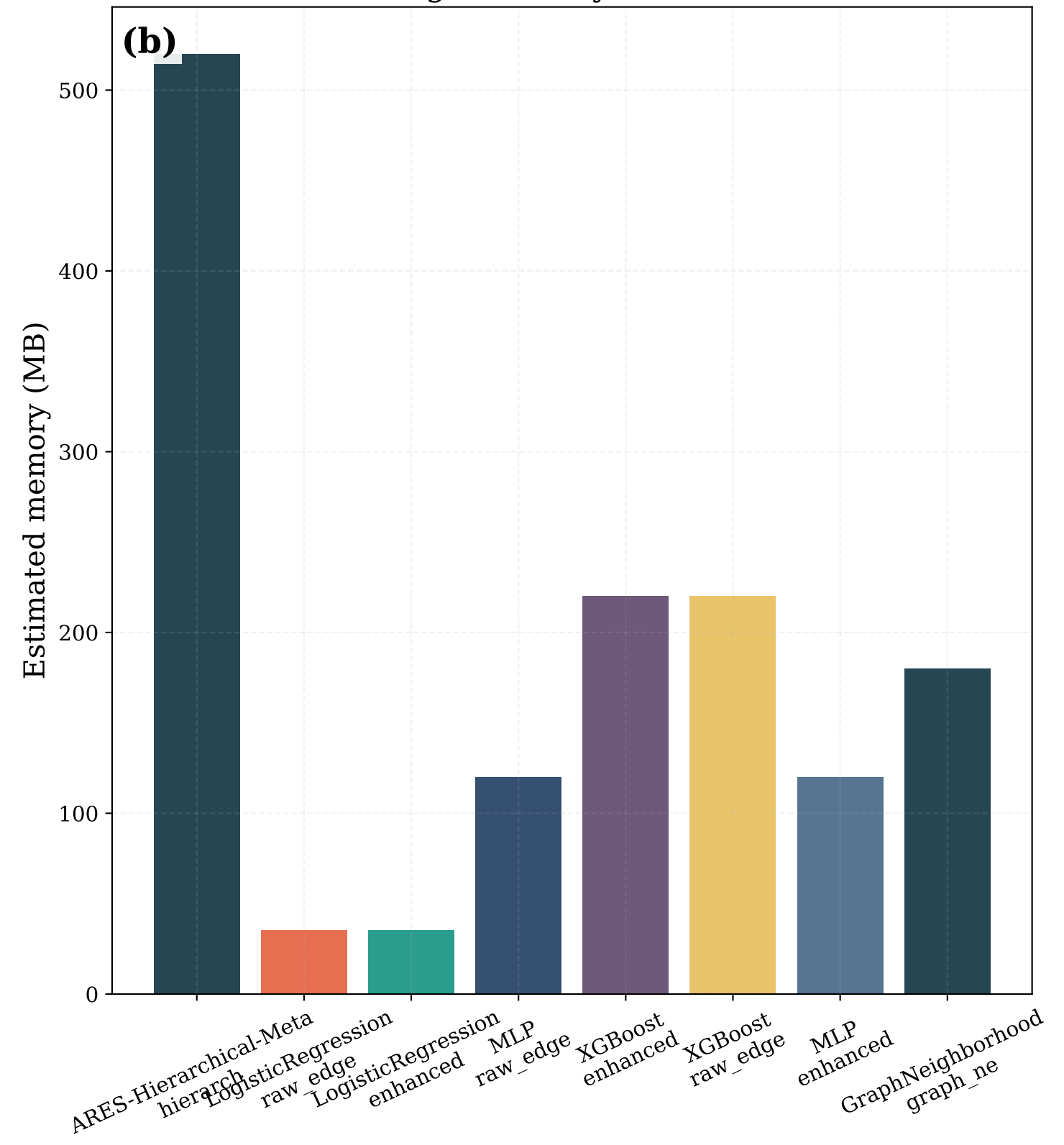
Edge memory estimate
