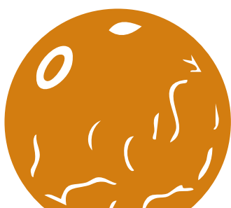
Mars
