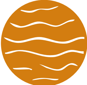
Venus
