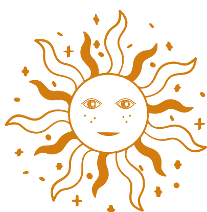
Sun
