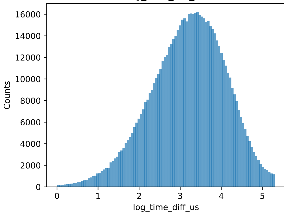
log_time_diff_us
