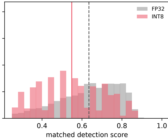
medium: shift -0.086
