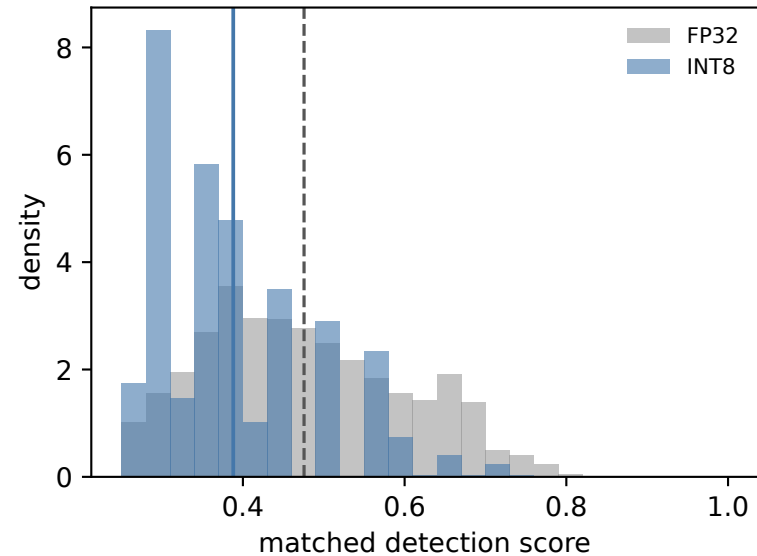
small: shift -0.088
