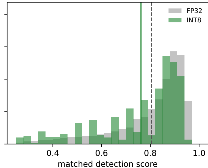
large: shift -0.043
