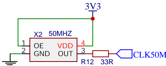
FPGA 50MHz crystal
