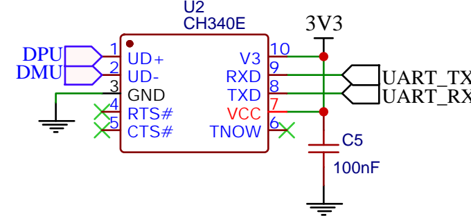
USB-UART
