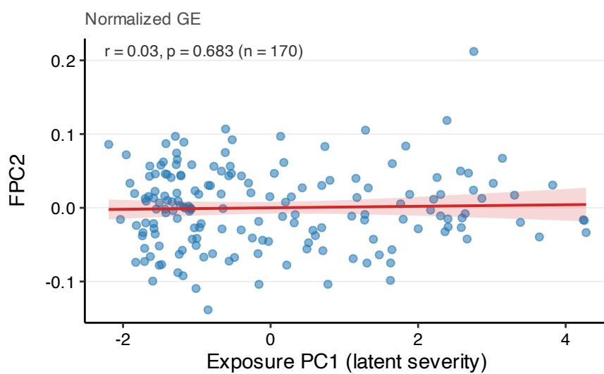
F. FPC2 vs. PC1
