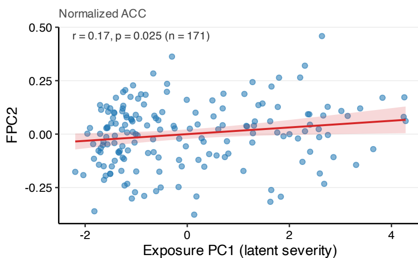
H. FPC2 vs. PC1
