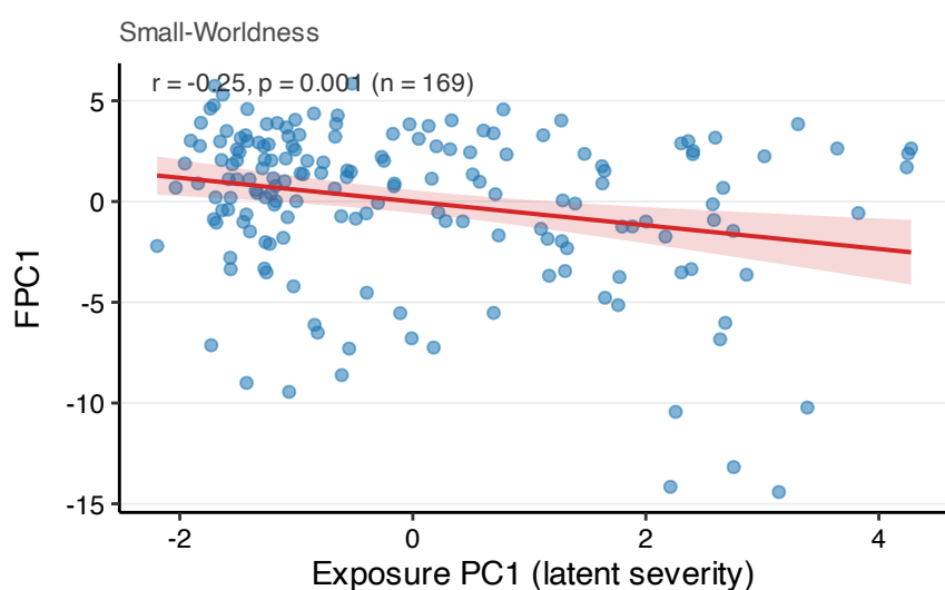
G. FPC1 vs. PC1
