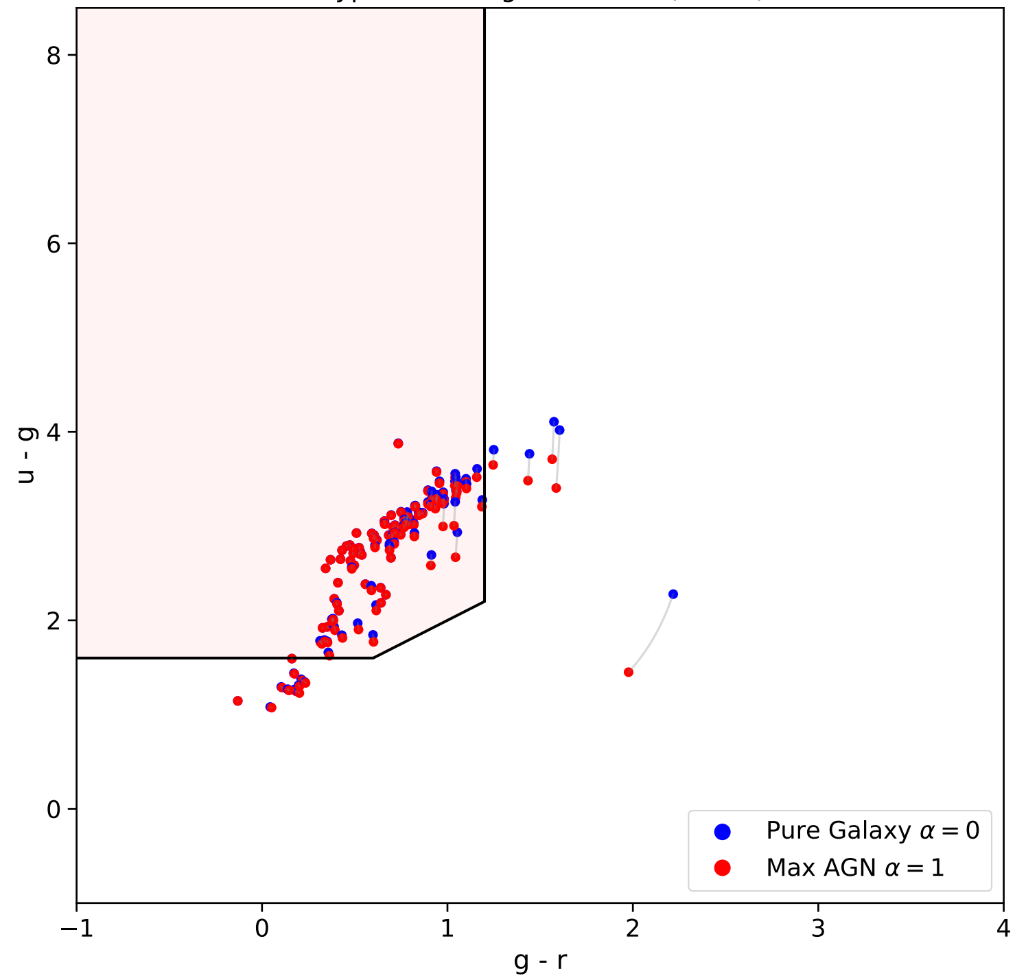
Type 2 AGN ugr Evolution (z=3.0)
