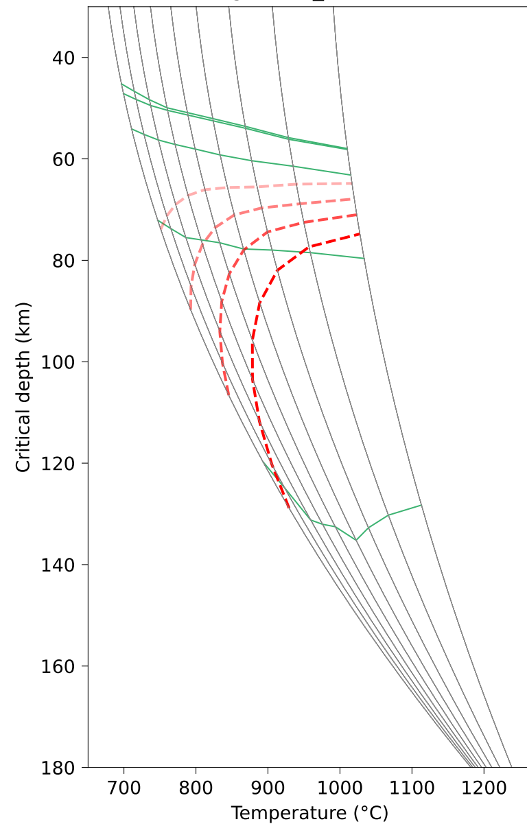
gulcher_venus
