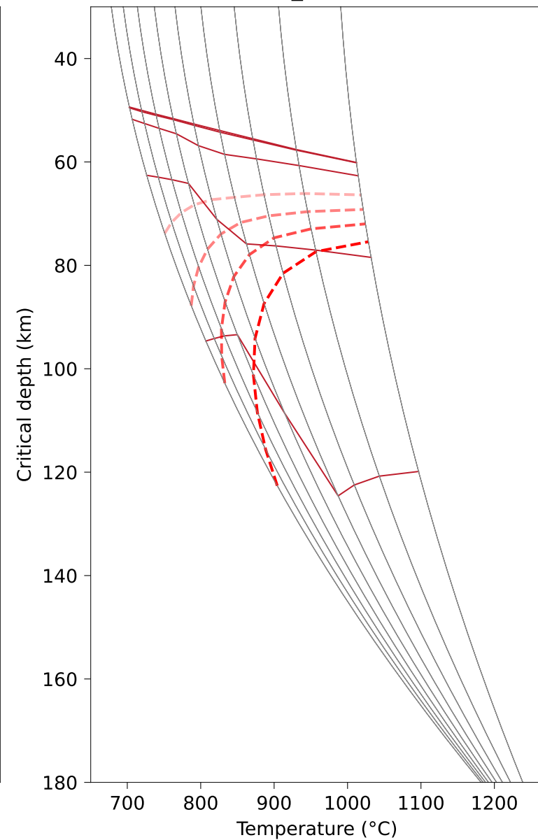
ito_basalt
