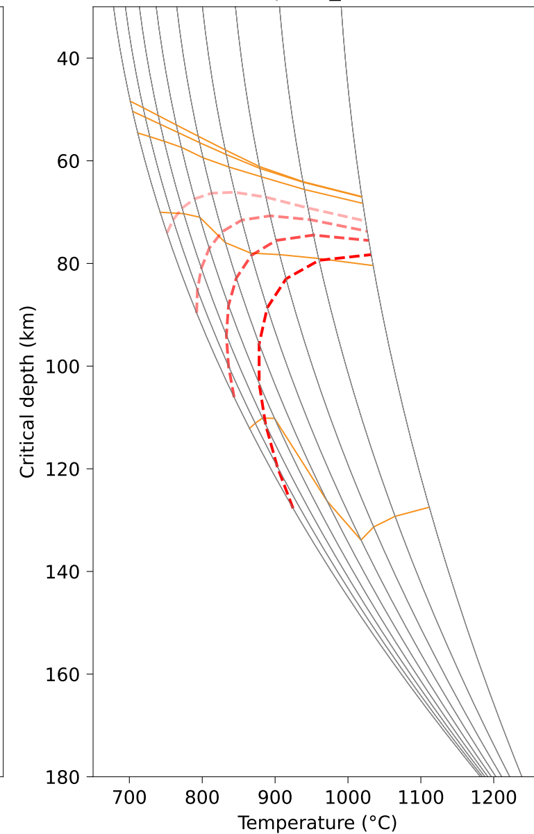
semprich_basalt
