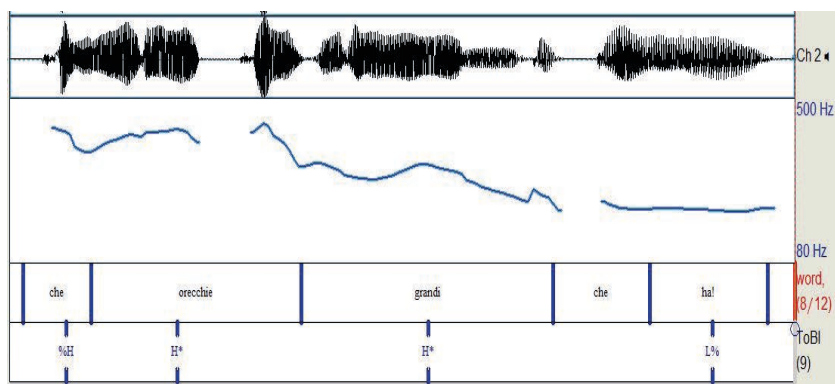
Figura 4. Forma d'onda, curva di f0 e trascrizione ToBI dell'enunciato esclamativo Che orecchie grandi che ha! prodotto da una locutrice di Cosenza
