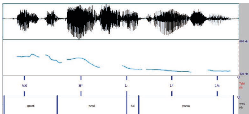
Figura 3. Forma d'onda, curva di f0 e trascrizione ToBI dell'enunciato esclamativo Quanti pesci hai preso! prodotto da una locutrice di Cosenza (fonte: Sorianello, 2011: 316).
