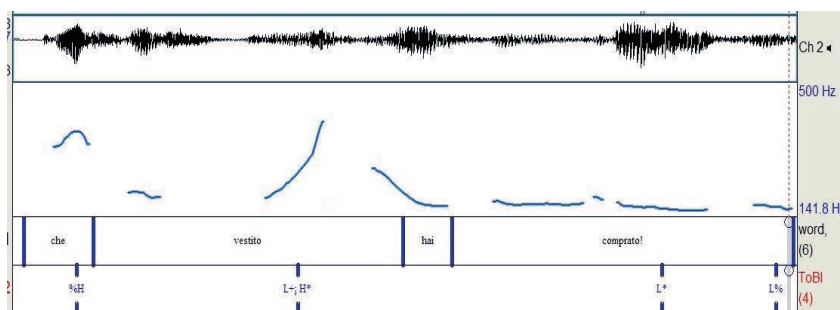
Figura 1. Forma d'onda, curva di f_0 e trascrizione ToBI dell'enunciato esclamativo Che vestito hai comprato! prodotto da una locutrice di Bari (esclwh-3-B_f-03).
