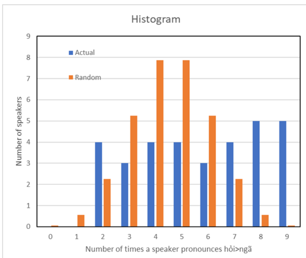
Hình 16. Cột xanh: Histogram số lần n mỗi người đọc hỏi > ngã. Cột cam: histogram cho trường hợp giả định kết quả hoàn toàn ngẫu nhiên, không ai phân biệt (phân phối nhị thức (binomial)).
