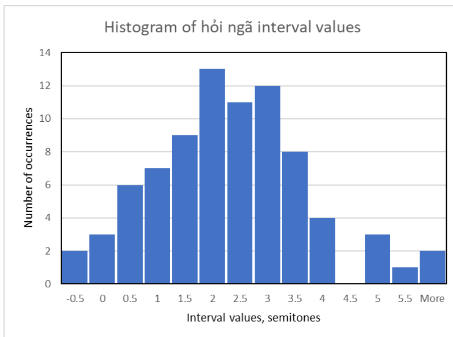
Hình 18. Phân phối quãng cách hỏi ngã trong 10 giọng phân biệt rõ ràng nhất.
