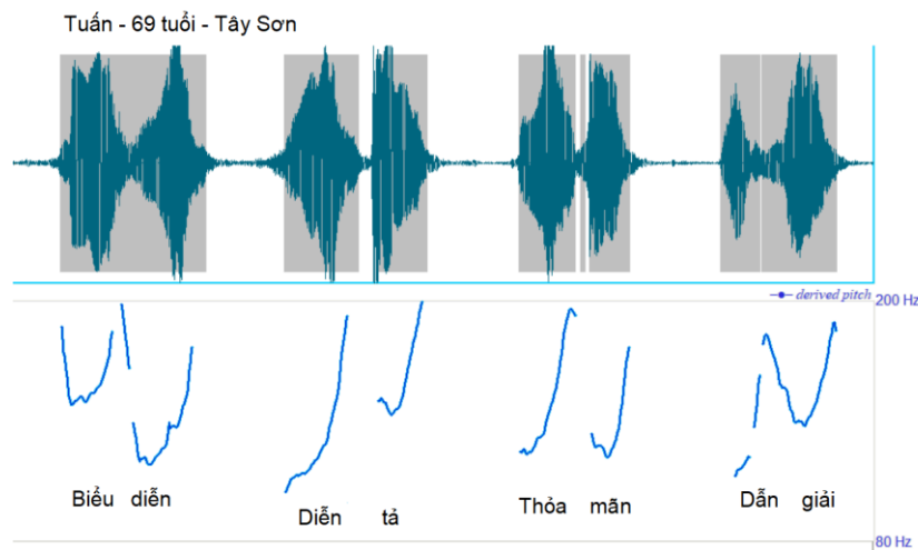
Hình 6. Độ cao (pitch contour) bốn chữ kép, (ông Tuấn, 69 tuổi, Tây Sơn). Chi tiết kỹ thuật như trên.
