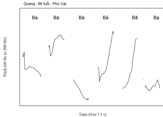
Hình 2. Đường nét độ cao (pitch contour) “ba bá bà bả bã bã bạ” (ông Quang, 66 tuổi, Phù Cát) dùng Praat. Pitch analysis parameters: raw autocorrelation method with floor 60 Hz, ceiling 200 Hz, silence threshold 0.1, voicing threshold 0.4, octave cost 0.1, octave jump cost 1.0, voiced / unvoiced cost 0.14.
