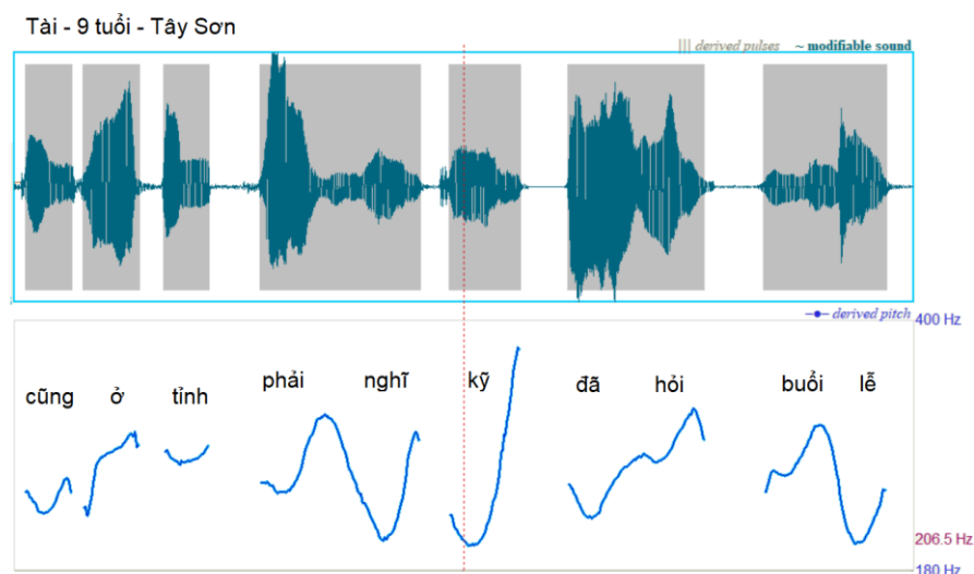
Hình 10. Độ cao (pitch contour) các dấu hỏi ngã trong một câu nói (em Tài, 9 tuổi, Tây Sơn). Chi tiết kỹ thuật như trên.
