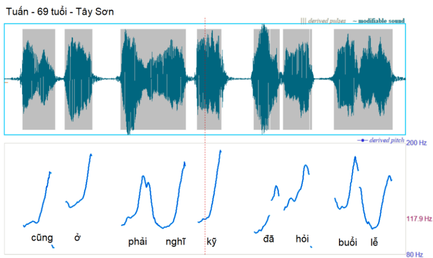
Hình 7. Độ cao (pitch contour) các dấu hỏi ngã trong một câu nói (ông Tuấn, 69 tuổi, Tây Sơn). Chi tiết kỹ thuật như trên.
