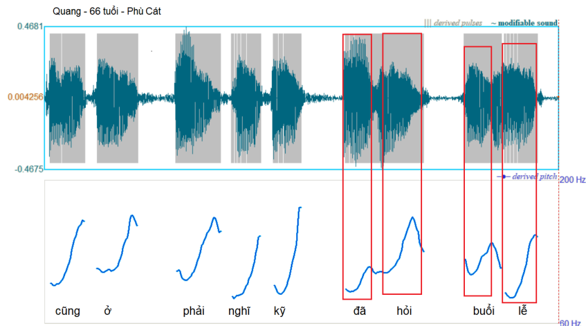
Hình 4. Độ cao (pitch contour) các dấu hỏi ngã trong một câu nói (ông Quang, 66 tuổi, Phù Cát). Chi tiết kỹ thuật như trên.
