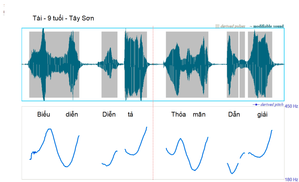
Hình 9. Độ cao (pitch contour) bốn chữ kép (em Tài, 9 tuổi, Tây Sơn). Chi tiết kỹ thuật như trên.
