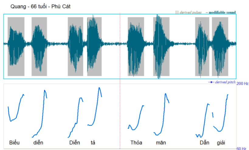
Hình 3. Độ cao (pitch contour) bốn chữ kép (ông Quang, 66 tuổi, Phù Cát). Chi tiết kỹ thuật như trên.
