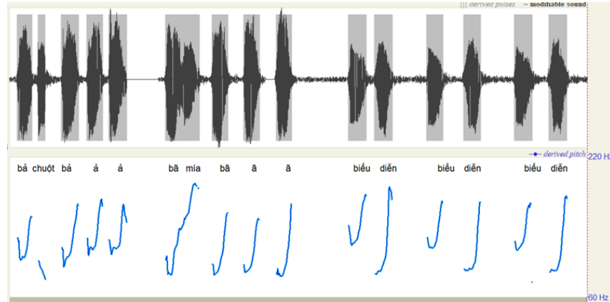
Hình 14. Biến đổi của thanh dấu trong một nhóm chữ.
