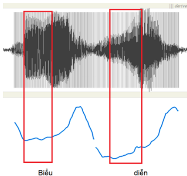
Hình 15. Dường cao độ của nửa âm đầu để so sánh hỏi và ngã.
