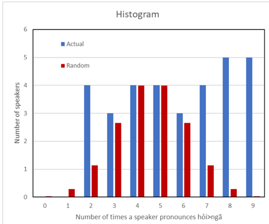
Hình 17. Cột xanh: biểu thị phân phối số lần n một người đọc hỏi>ngã. Cột đỏ: biểu thị phân phối cho nhóm không phân biệt (phân phối nhị thức với đỉnh ở n = 4-5 bằng số lần đo được).
