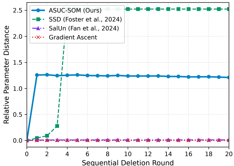
(b) Parameter Distance Drift \|\Delta\theta_t\|/\|\theta_0\|
