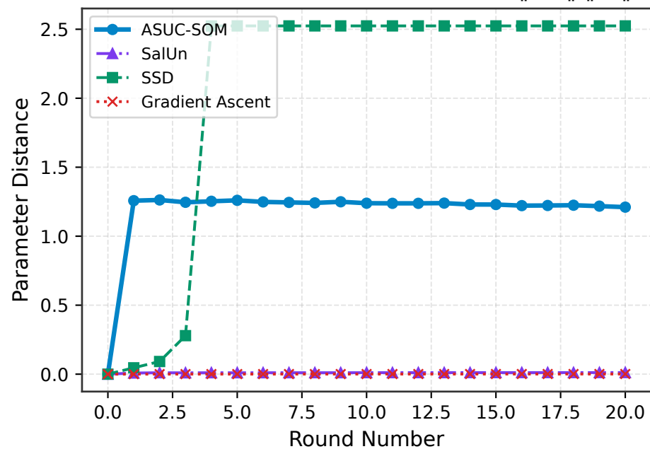
(d) Relative Parameter Distance \|\Delta\theta_t\|/\|\theta_0\|
