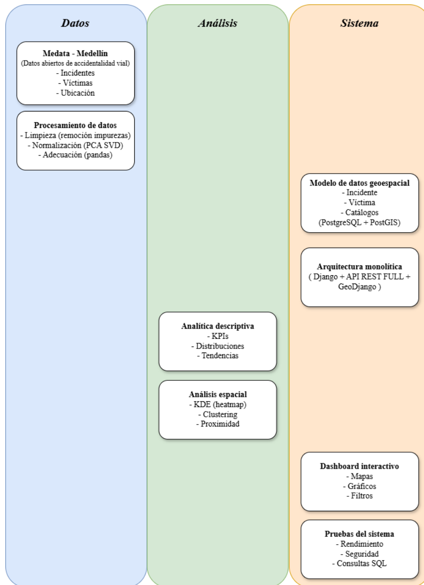
Fig. 6. DIAGRAMA DE METODOLOGÍA
