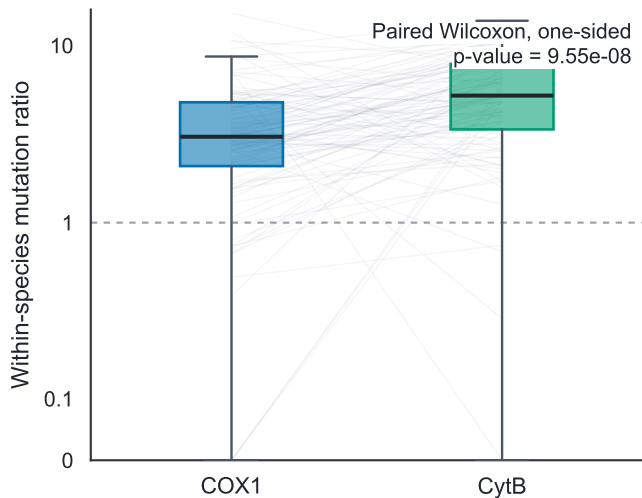
A C>T / G>A
