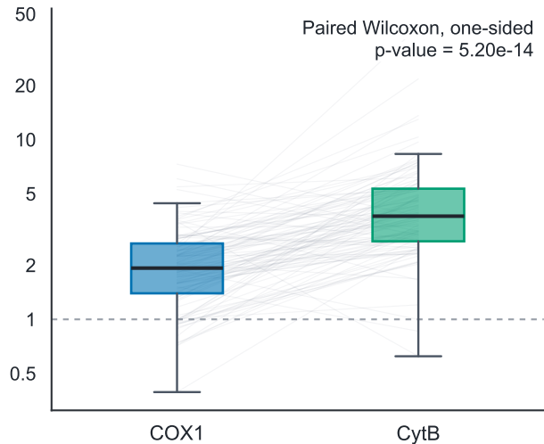
B A>G / T>C
