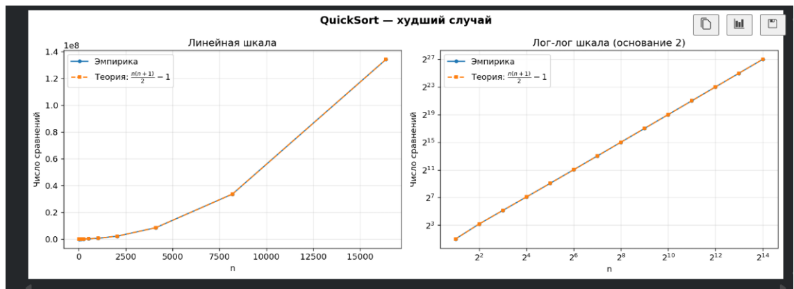
Рисунок 6 - Сопоставление эмпирики и теории для QuickSort
