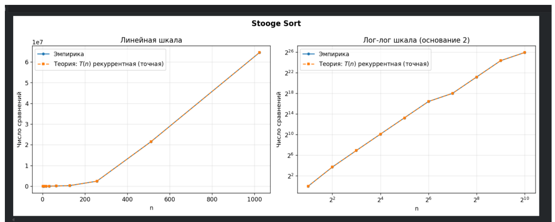
Рисунок Б.5 — Сопоставление эмпирических и теоретических данных для сортировки Студжа
