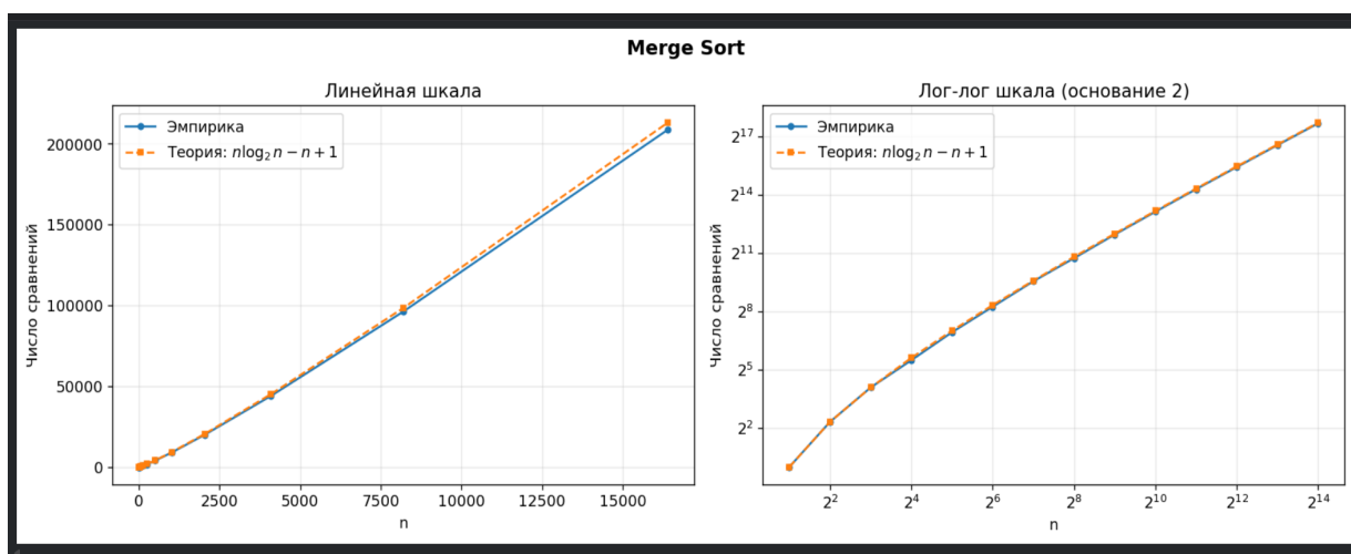
Рисунок Б.1 - Сопоставление эмпирических и теоретических данных для сортировки слиянием
