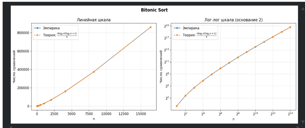
Рисунок 4 - Сопоставление эмпирического и теоретического числа сравнений для битонической сортировки
