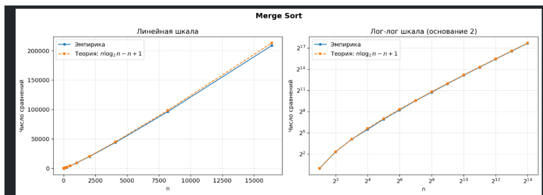
Рисунок 5 - Сопоставление эмпирики и теории для MergeSort
