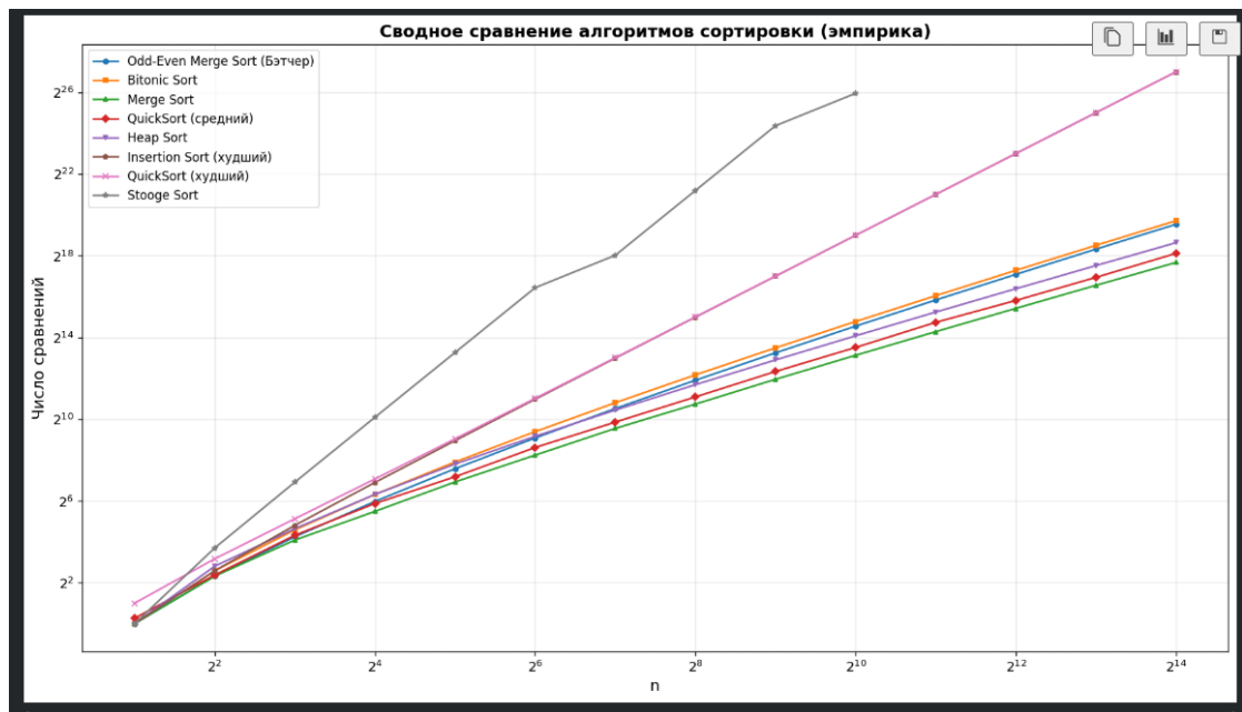
Рисунок 7 - Сводное сравнение алгоритмов сортировки по числу сравнений
