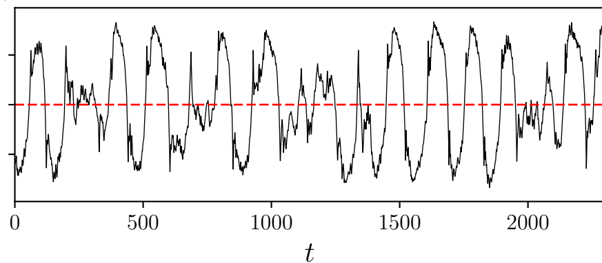
(d) Ra = 3 \cdot 10^7 inside iii - iv
