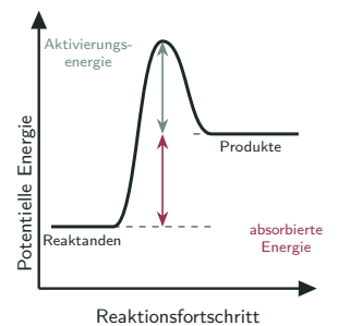
Endotherme Reaktion
