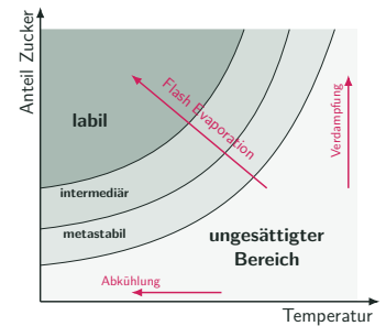
■ Abbildung 18: Schematische Darstellung des Zusammenhangs von Temperatur und Verdampfung auf die Kristallbildung in einer Saccharoselösung.
