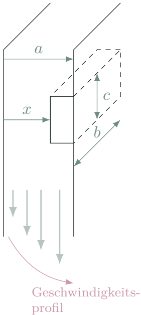
■ Abbildung 5: Modelldarstellung Geschwindigkeitsprofil. An der Wand ist Geschwindigkeit v = 0 und steigt parabelförmig an.
