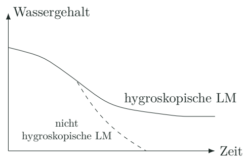
■ Abbildung 23: Trocknung von hygroskopischen und nicht-hygroskopischen Lebensmitteln
