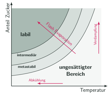
■ Abbildung 18: Schematische Darstellung des Zusammenhangs von Temperatur und Verdampfung auf die Kristallbildung in einer Saccharoselösung.
