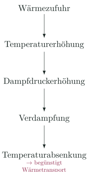
■ Abbildung 19: Trocknungsprozess
