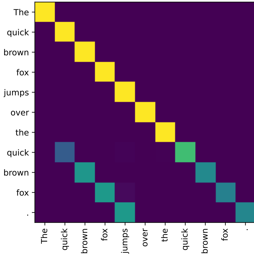
gpt2 L0H1
