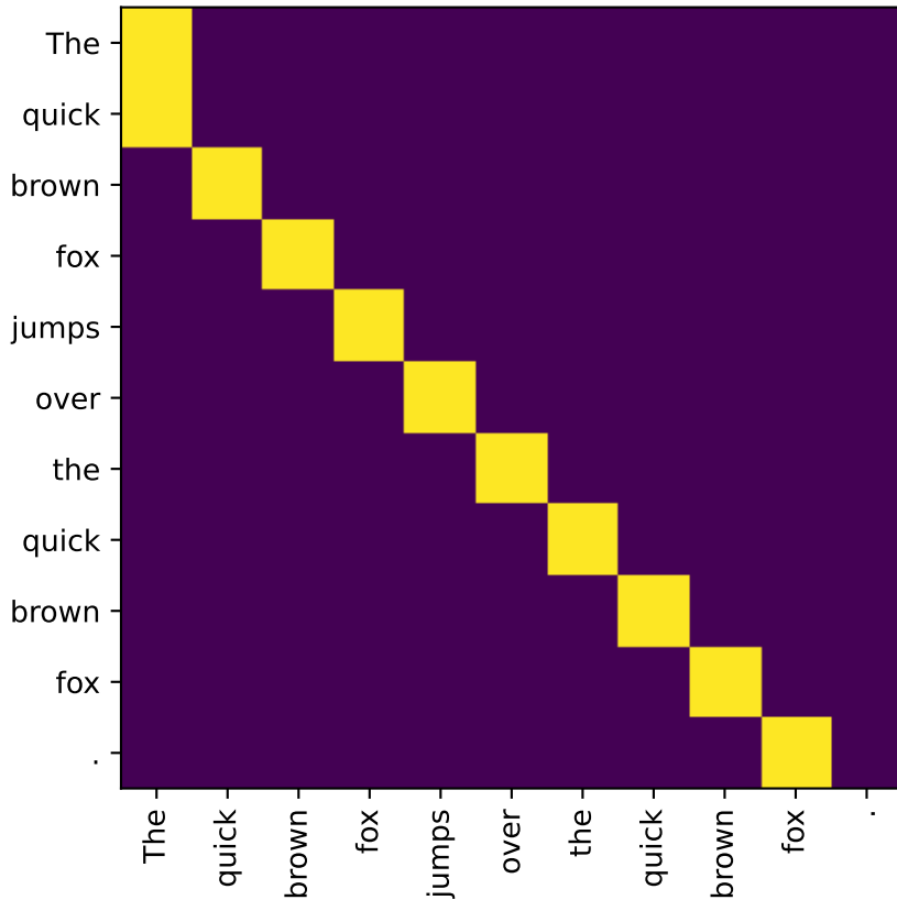
gpt2 L4H11
