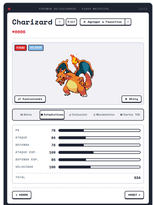
Figura 8. Pestaña Estadísticas.
