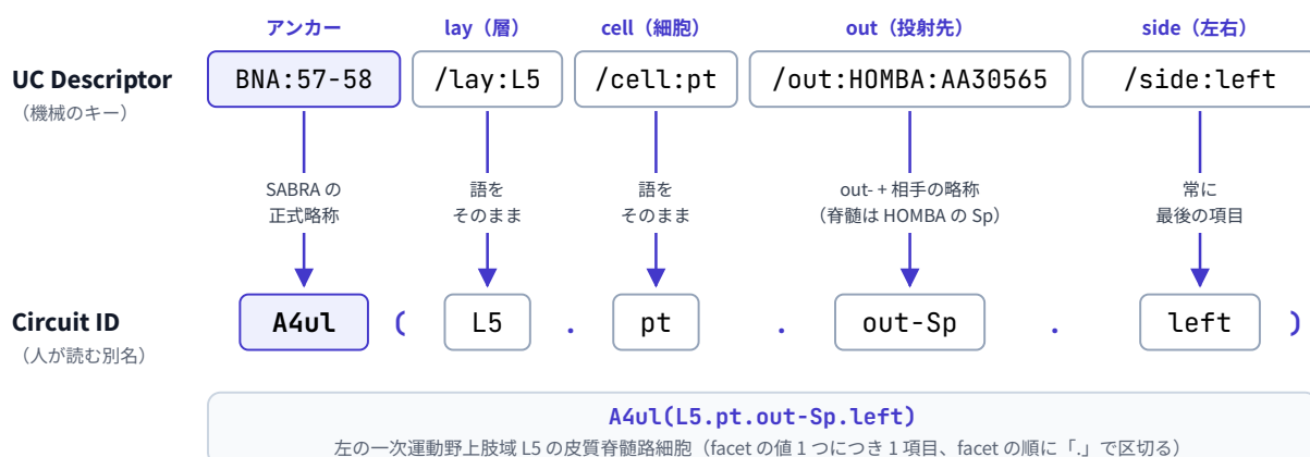
図 2.2 UC Descriptor から Circuit ID を組み立てる。前半はアンカーの正式略称、括弧の中は facet の値を順に並べたもの
