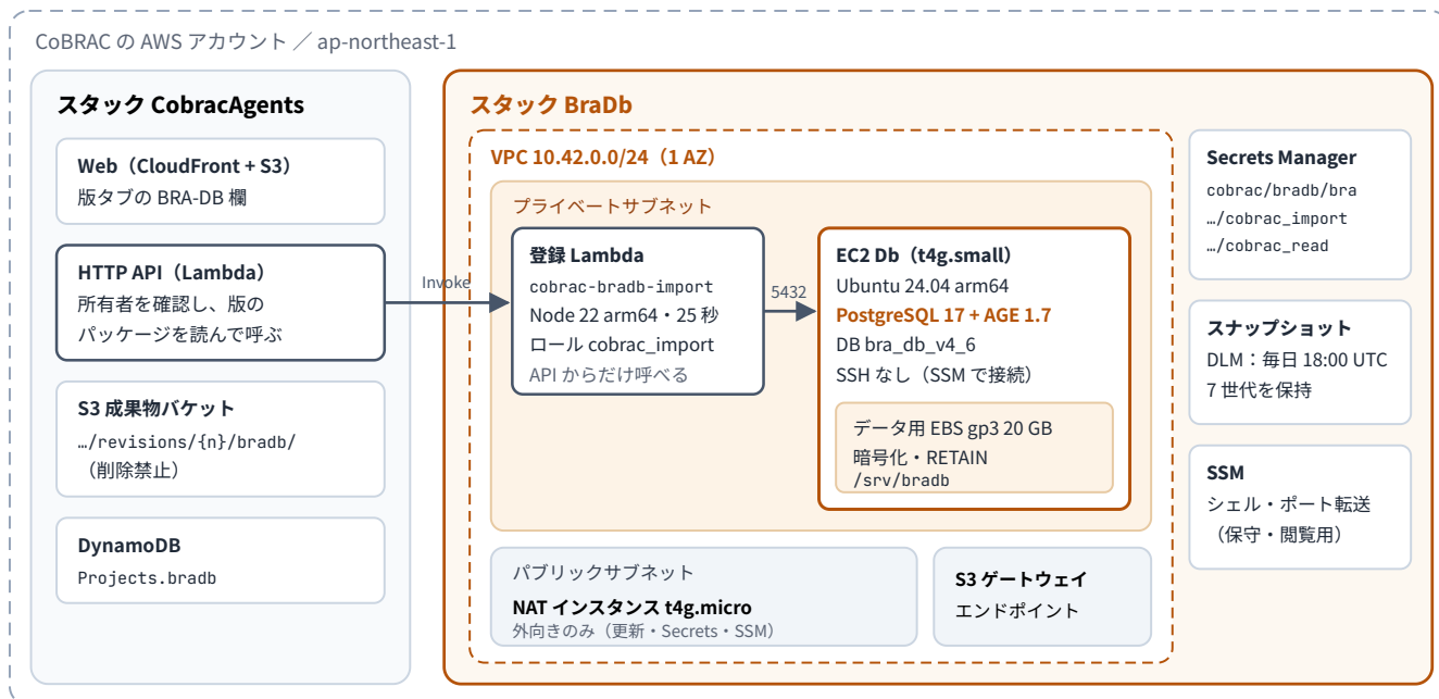
図 7.2 BRA-DB の AWS の構成。データベースは VPC のプライベートサブネットにあり、5432 番は登録 Lambda からしか受けない
