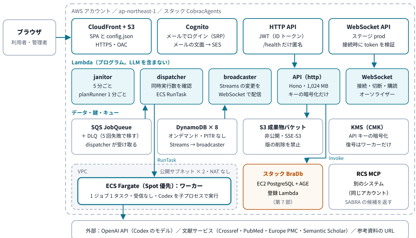
図 8.2 AWS の構成。Lambda とワーカーはどちらも LLM を含まないプログラムで、エージェントはワーカーが起動する Codex を通して OpenAI API で推論する
