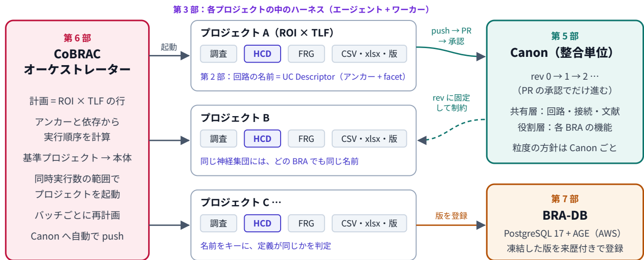
図 1.1 仕組みの関係。各プロジェクトの中では、ハーネス（第3部）がBRAを作る。オーケストレーター（第6部）は多数のプロジェクトを起動する。各プロジェクトはUC Descriptor（第2部）で回路に名前を付け、Canon（第5部）で定義をそろえ、凍結した版をBRA-DB（第7部）に登録する。全体を支えるシステムは第8部、セキュリティと費用は第9部
