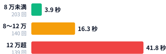
1 回の応答の固定の待ち時間（秒）
